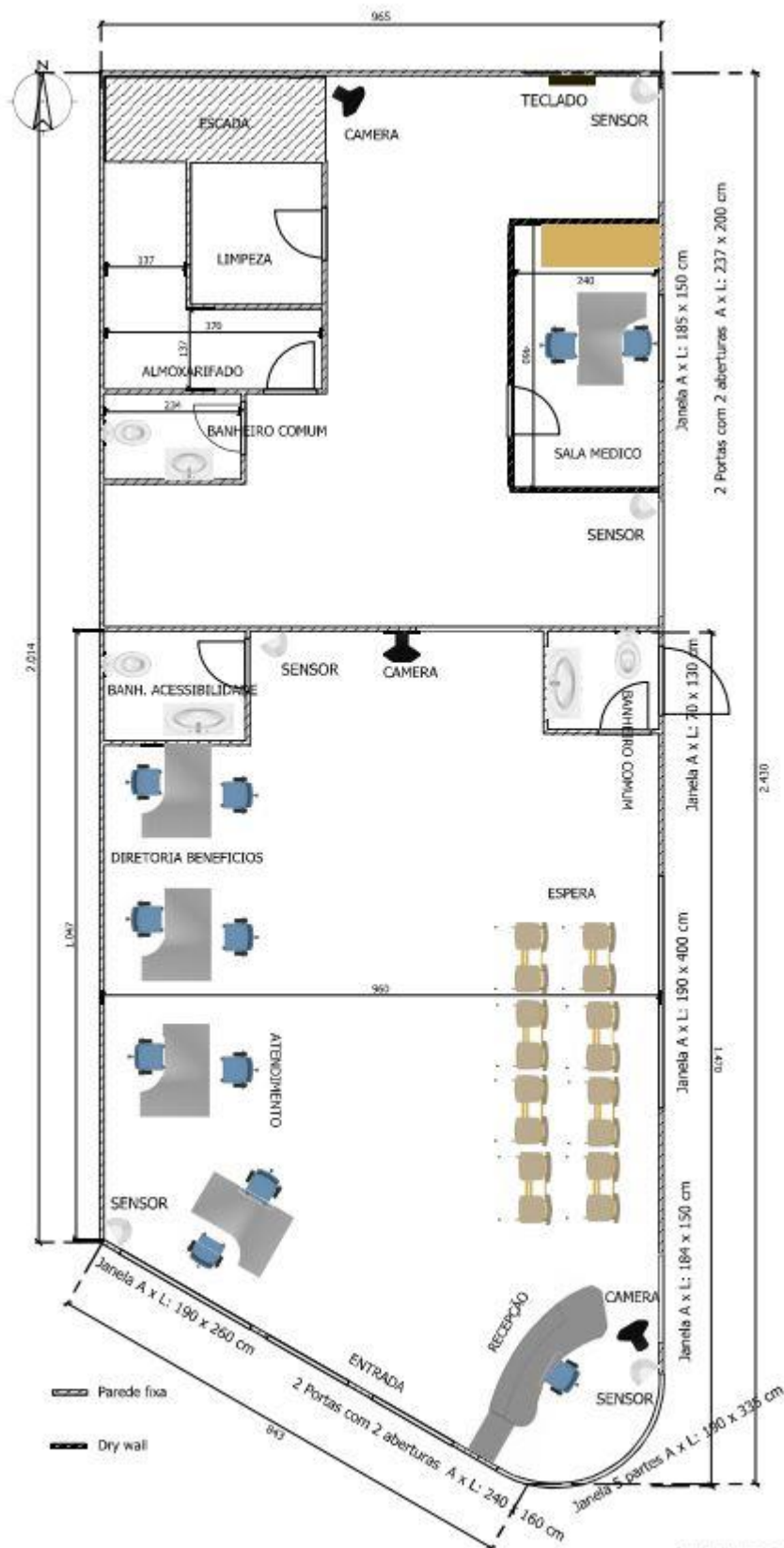
PLANTA TERREO
